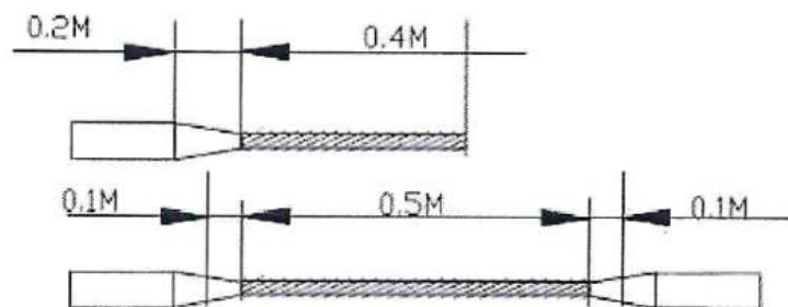
Рис. 6. Соединение медных жил одножильного кабеля с изоляцией
